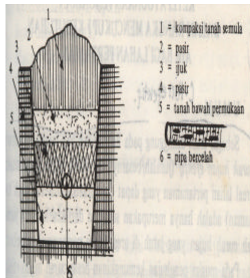
Gambar 47. Sketsa pembuangan drainase
