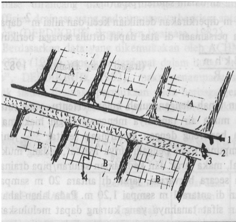
Gambar 44 Sketsa lahan pertanian dengan saluran irigasi dan saluran drainase searah.
