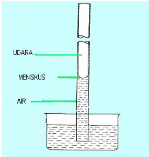
Gambar 12 Peristiwa kapilaritas
