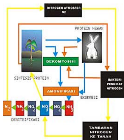
Gambar 14. Peredaran nitrogen
