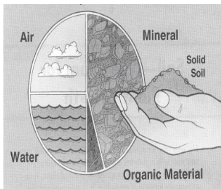
Gambar 35 Perbandingan volumetrik dari komposisi tanah
