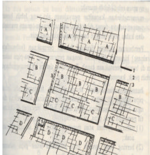
Gambar 45 Sketsa lahan pertanian dengan penurunan pangkal dan topografi teratur dengan saluran drainase sejajar
