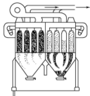
Gambar 11.9 Pengendap siklon
