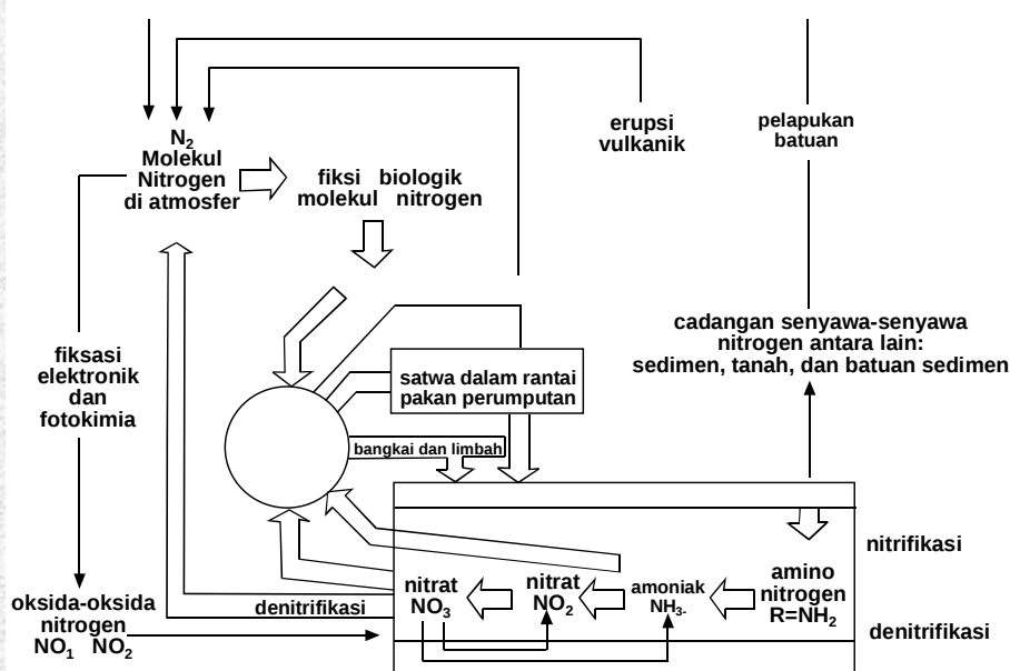
Gambar 10.9 Daur nitrogen (Sumber: Dasar-Dasar Ekologi , 2003)
