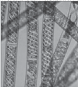
Gambar 5.8 Spirogyra (Sumber: www.biltek.tubitek.gov.tr )
