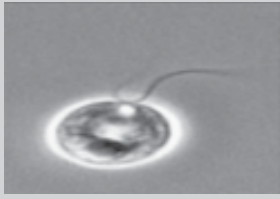
Gambar 5.7 Chlamydomonas merupakan Chlorophyta bersel satu yang dapat bergerak. (Sumber: www.biltek.tubitek.gov.tr )
