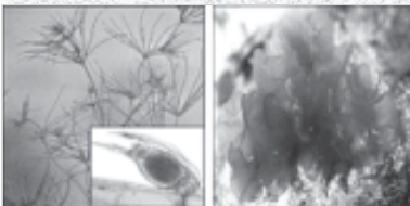
Gambar 5.9 Chara dan Ulva yang merupakan Chlorophyta berbentuk lembaran. (Sumber: www.biltek.tubitek.gov.tr )
