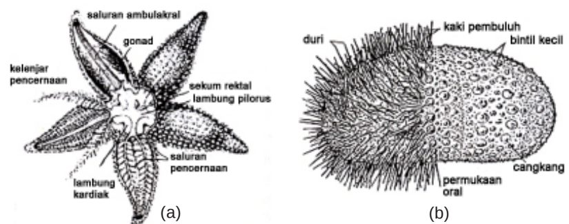
Gambar 9.25 Berbagai hewan Echinodermata
