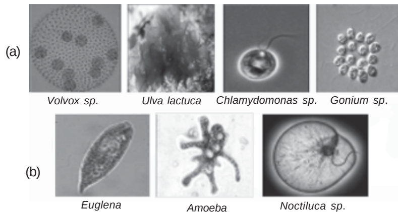
Gambar 5.3 (a) Protista mirip tumbuhan dan (b) Protista mirip hewan (Sumber: www.biltek.tubitek.gov.tr )
