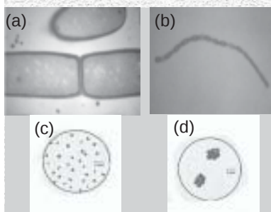
Gambar 4.2 Bentuk-bentuk bakteri: (a) Diplococcus bacillus ; (b) Spirillum ; (c) Stephylococcus ; (d) Sarcina ventriculi . (Sumber: Pelczar, M.J., dan Chan, 1986 dan Http://www.monera.org )
