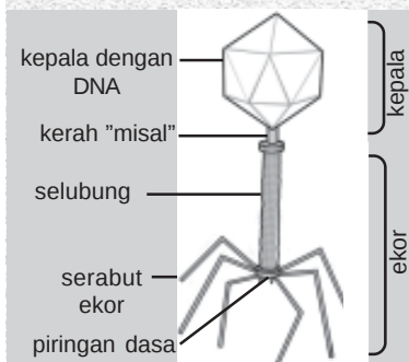
Gambar 3.4 Struktur virus bakterifag T2 (Sumber: Encarta Encyclopedia , 2006)
