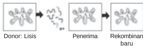
Gambar 4.6 Transformasi (Sumber: www.e-dukasi.net )
