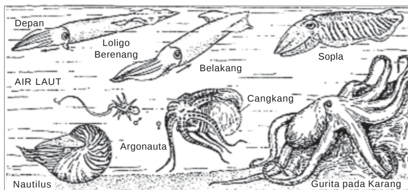
Gambar 9.19 Cephalopoda (Sumber: Zoologi Dasar, 1989)
