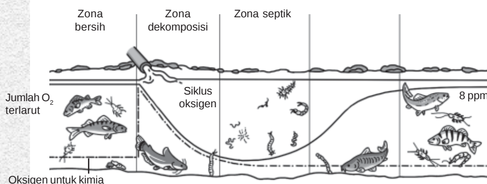
Gambar 11.3 Dampak zat pengikat oksigen udara dalam air (Sumber: Kesehatan Lingkungan , 2005)
