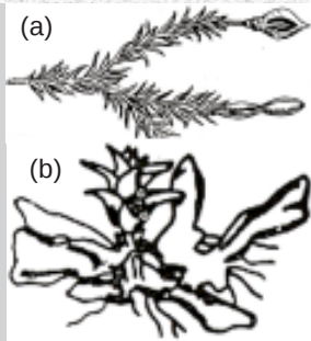
Gambar 8.3 (a) Andreaea rupestris ; (b) Sphagnum (Sphagnaceae)
