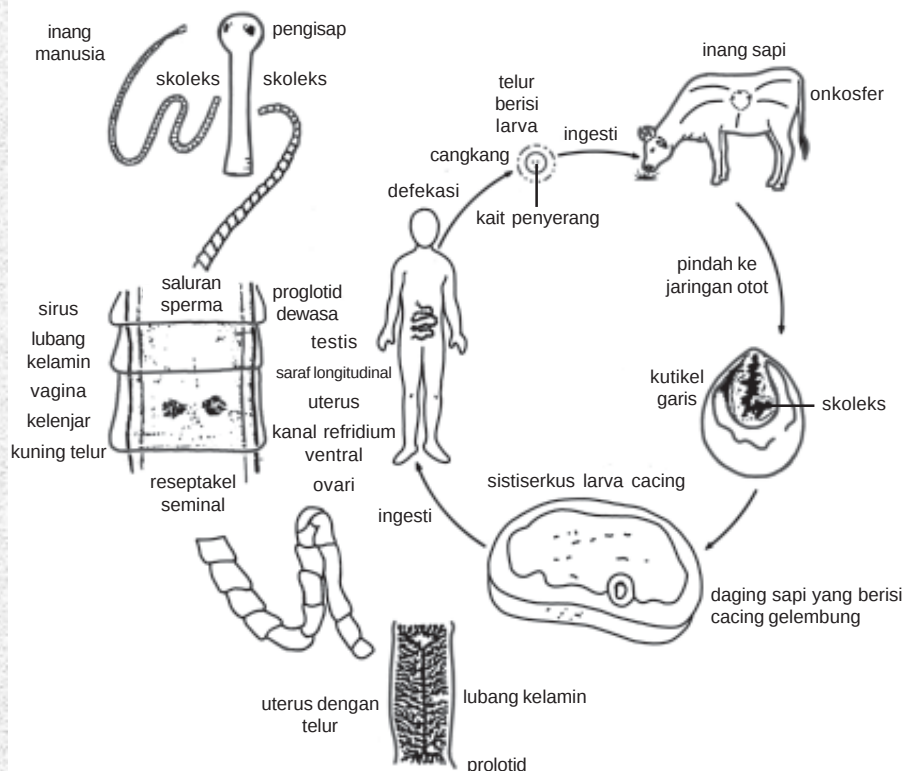
Gambar 9.10 Daur hidup cacing pita T. saginata (Sumber: Zoologi Dasar, 1989)
