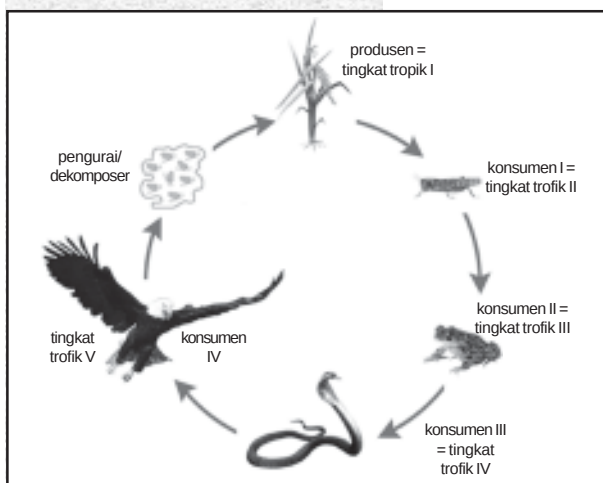
Gambar 10.6 Saling ketergantungan antara produsen, konsumen, dan dekomposer (Sumber: Koleksi pribadi)
