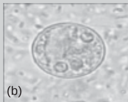
Gambar 5.17 (a) Amoeba dan (b) Entamoeba (Sumber: www.e-dukasi.net )
