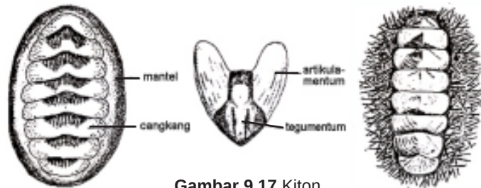
Gambar 9.17 Kiton (Sumber: Zoologi Dasar, 1989)
