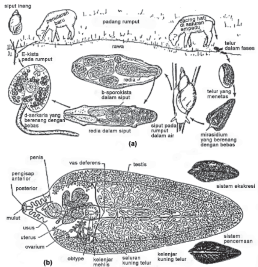
Gambar 9.9 Fasciola hepatica : (a) Daur hidup dan (b) Sistem reproduksi (Sumber: Zoologi Dasar, 1989)
