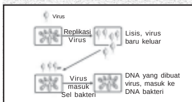
Gambar 4.8 Transduksi (Sumber: www.e-dukasi.net )
