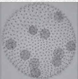
Gambar 5.10 Volvox (Sumber: Taksonomi tumbuhan , 2005)
