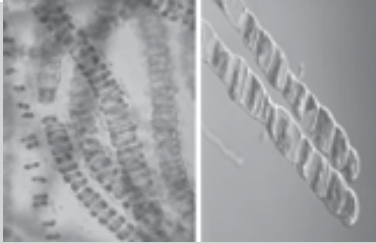
Gambar 5.5 Ulothrix zonata merupakan salah satu kelompok Ulothrix sp. (Sumber: www.dipbot.unict.it dan www.nies.go.jp )
