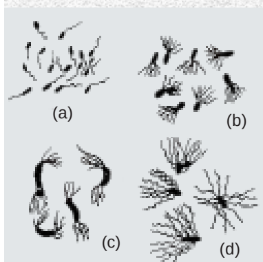
Gambar 4.3 Jenis-jenis bakteri berdasarkan jumlah flagel: (a) monorik; (b) lofotrik; (c) subpolar; (d) peritrik. (Sumber: Pelczar, M.J. dan Chan, 1986 dan Http://www.monera.org )
